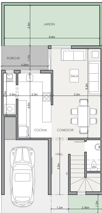
PLANTA BAJA: 52,46 m 2
