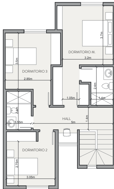
PLANTA ALTA: 63,91 m 2
